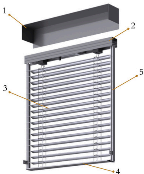
1 باکس محافظ سازه قابل اجراء بصورت توکار و روکار
